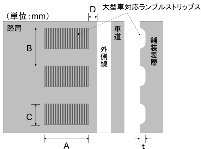
図6-2. ランブルストリップス詳細図
