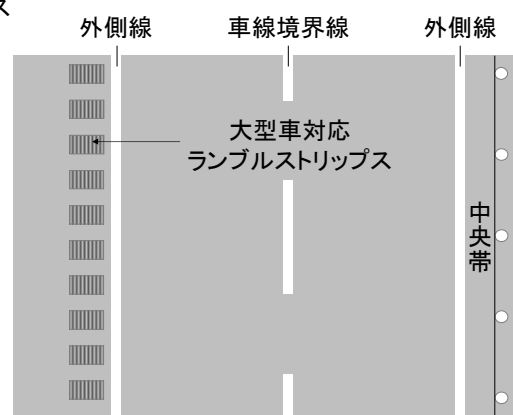
図6-3. ランブルストリップス設置位置
