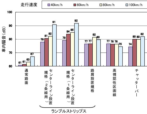
図 5-3. 車内騒音測定結果
