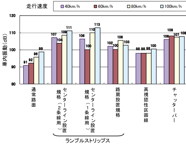
図 5-4. 車内振動測定結果
