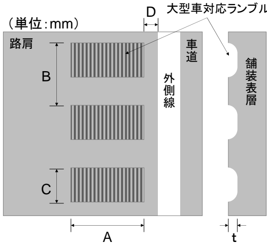
図6-2. ランブルストリップス詳細図
