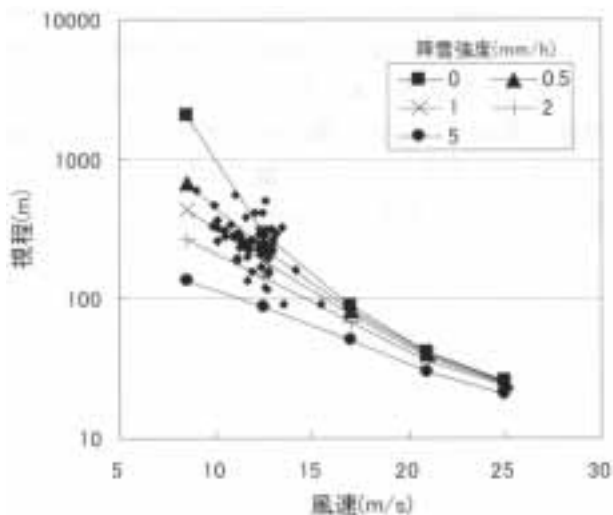
図 6 高さ 1.6m における視程の計算値と実測値の比較( :2000 年 12 月 22 日 03:00~04:00 の実測値。 :降雪強度 = 0mm/h。 :降雪強度 = 0.5mm/h。 x :降雪強度 = 1mm/h。 + :降雪強度 = 2mm/h。 :降雪強度 = 5mm/h の場合の計算値)
