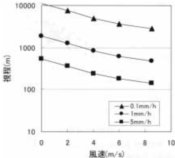
図8 降雪成分のみの場合における視程の計算値 ( : 降雪強度 = 0.1mm/h、 : 降雪強度 = 1mm/h、 : 降雪強度 5mm/h の条件で、風速を 0m/s、2m/s、4m/s、6m/s、8.4m/s と変化させた)
