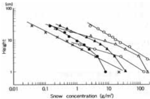
図3 石狩での飛雪濃度の垂直分布 12)
