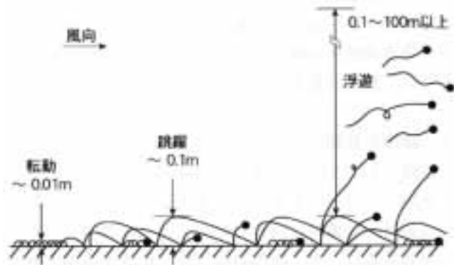
図1 吹雪の運動形態 5)
