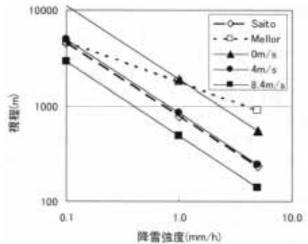
図9 風速が 8.5m/s 未満の場合の降雪強度と視程の関係[ : 斎藤 10) が、自らの実測値から求めた式に基づく計算値。 : 斎藤 10) が Mellor 9) の実測値から求めた式に基づく計算値。 : 本研究で求めた式に基づく計算値(風速 = 0m/s)。 : 本研究で求めた式に基づく計算値(風速 = 4m/s)。 : 本研究で求めた式に基づく計算値(風速 = 8.4m/s).]
