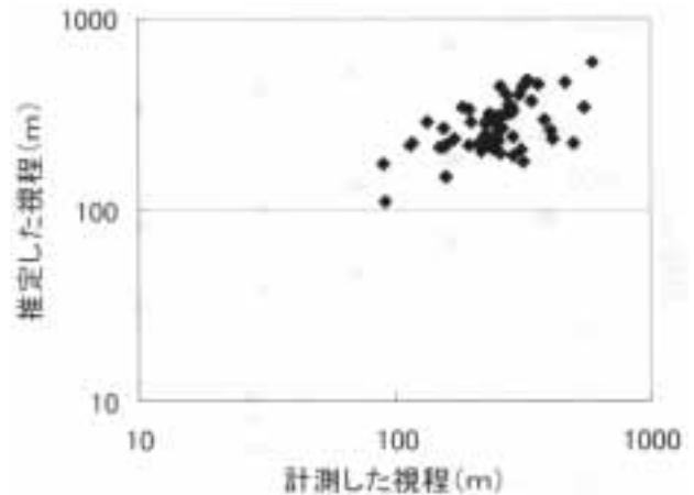
図 7 降雪強度を 0.5mm/h と仮定して計算した視程と実測値との比較
