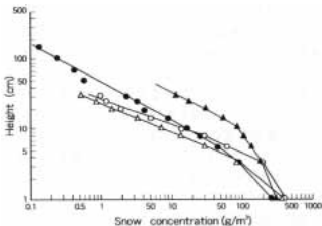
図4 ワイオミングでの飛雪濃度の垂直分布 18)
