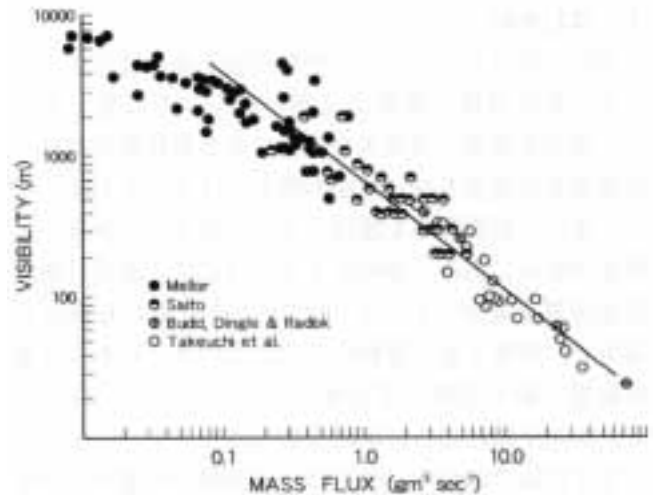
図2 視程と飛雪流量の関係 13) (両対数のグラフで、両者は直線近似できる)
